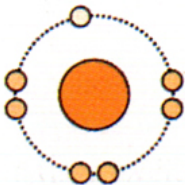
Volný radikál
