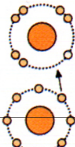
Molekula
