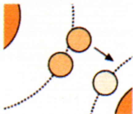
Volný radikál
